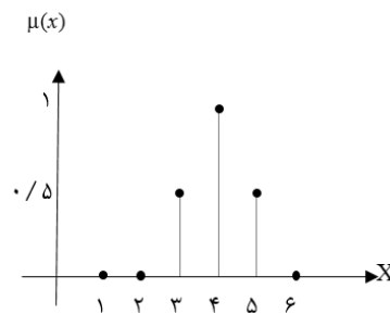
شکل ۱۵-۱۰. نمودار تابع عضویت مجموعه فازی \tilde{A}
